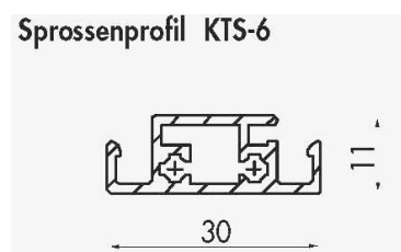
Sprossenprofil
