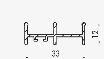
3-fach Bodenschiene M3B-6
