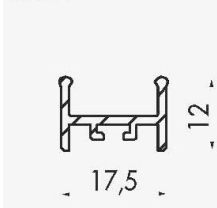
2-fach Bodenschiene M2B-6
