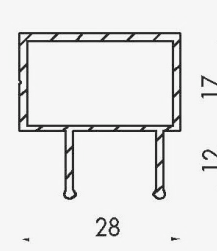
2-fach Rahmenprofil M2R-6
