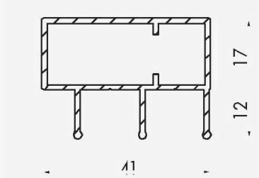
3-fach Rahmenprofil M3R-6
