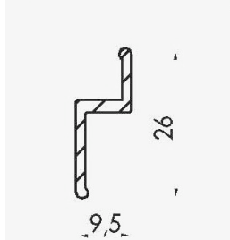
1-fach Boden- und Deckenschiene M1F-6
