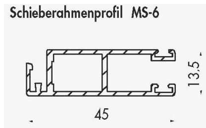
Rahmenprofil
